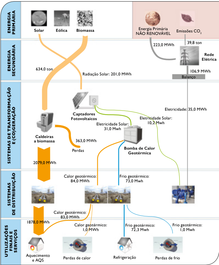
Figura 9 Diagrama Sankey do Sistema de Olot.
