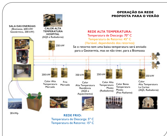
Figura 5 Esquema de funcionamento da rede em modo verão (Fonte: AIGUASOL).
