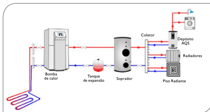
Figura 3 Esquema do princípio da Bomba de Calor Geotérmica (Fonte: GNS).
