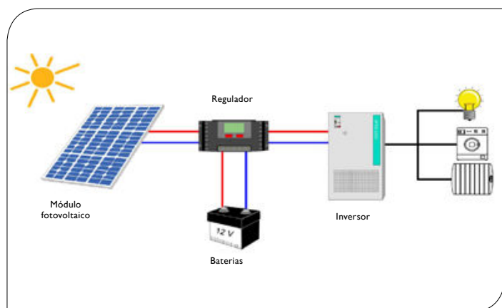
Figura 4 Esquema de princípio fotovoltaico (Fonte: GNS).
