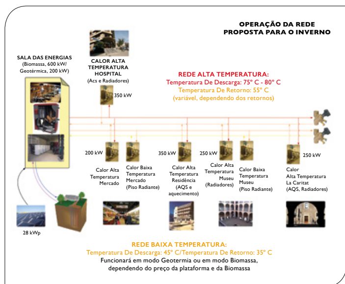
Figura 6 Esquemas de funcionamento da rede em modo inverno (Fonte: AIGUASOL).
