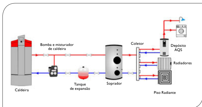
Figura 2 Esquema de princípio Caldeira de Biomassa (Fonte: GNS).
